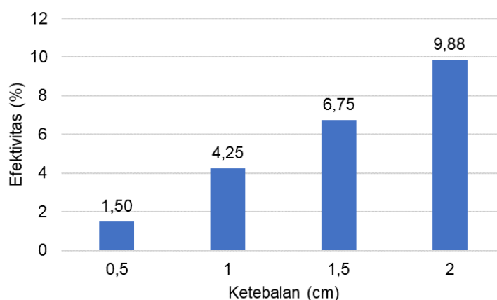
Gambar 4 Nilai efektivitas reduksi kebisingan saat sumber bunyi pada jarak 75 cm
