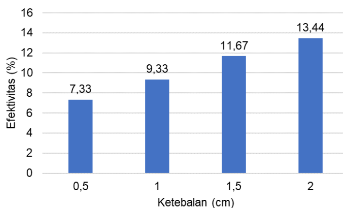
Gambar 2 Nilai efektivitas reduksi kebisingan saat sumber bunyi pada jarak 25 cm
