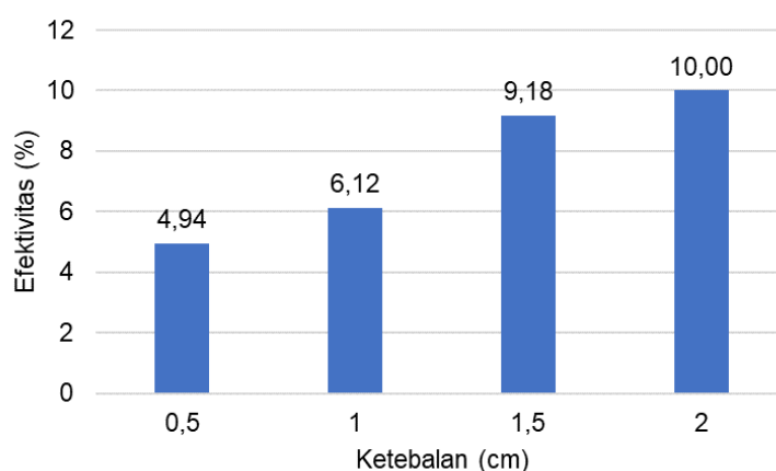
Gambar 3 Nilai efektivitas reduksi kebisingan saat sumber bunyi pada jarak 50 cm
